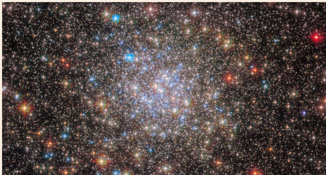
Estrelas de diversas cores no aglomerado globular NGC6355, na Via Láctea, registradas pelo Telescópio Hubble. Crédito: ESA/Hubble & NASA, E. Noyola, R. Cohen
